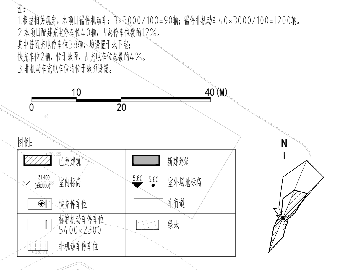
总平面图 1:500
