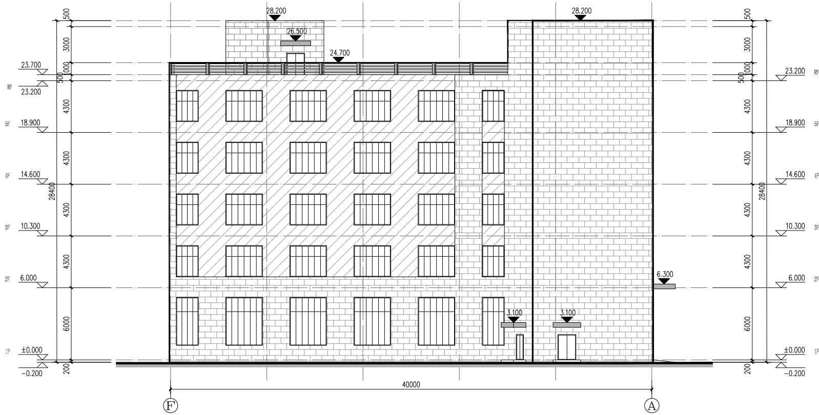
厂房五 ⑥-①轴立面图 1:150
