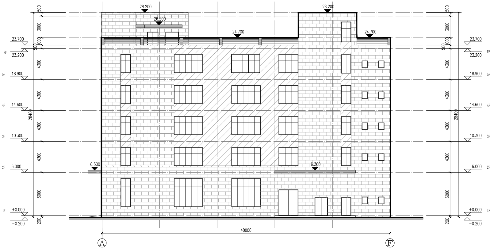
厂房五 ①-⑤轴立面图 1:150
