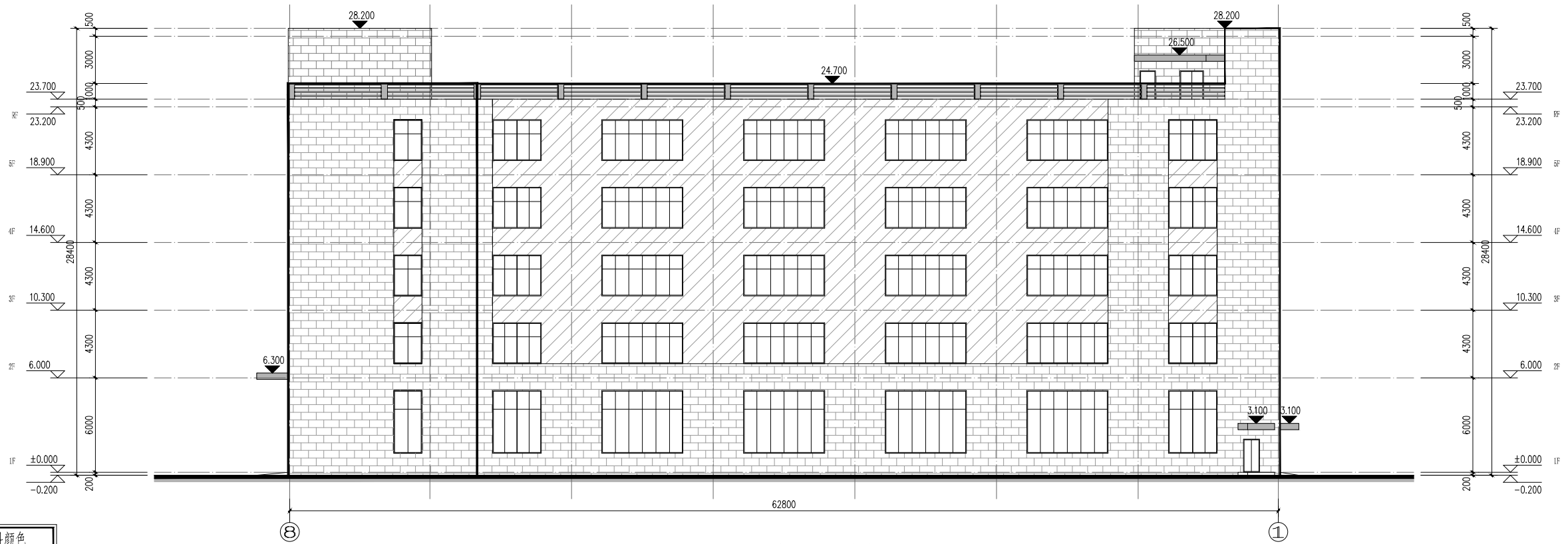
厂房五 ⑧-①轴立面图 1:150
