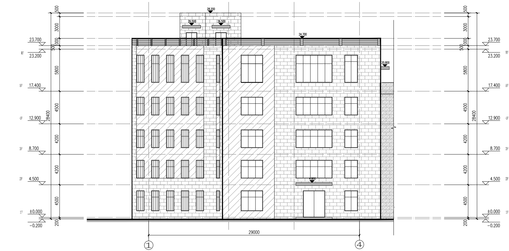
厂房三 ①-④轴立面图 1:150
