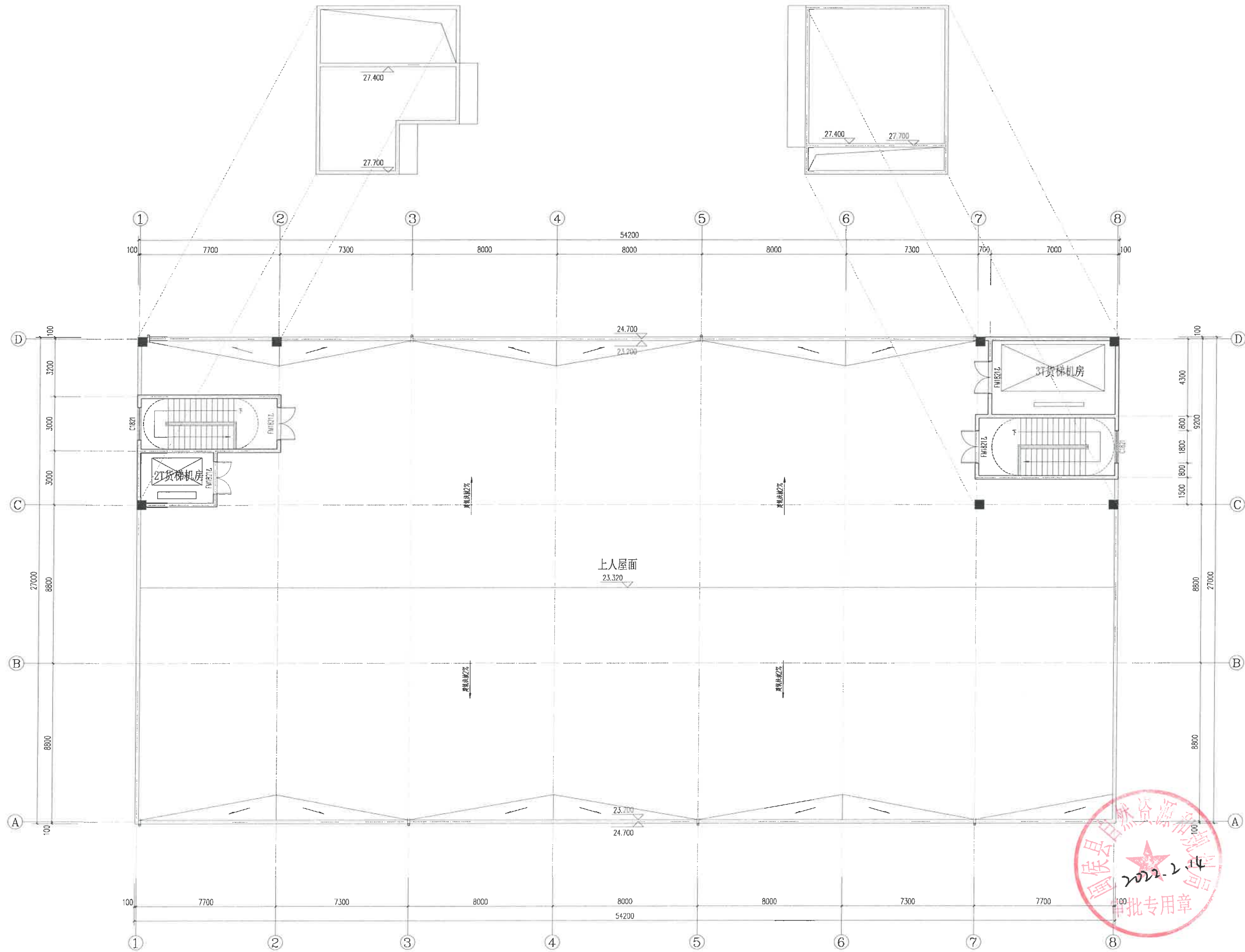
屋顶层平面图 1:100
