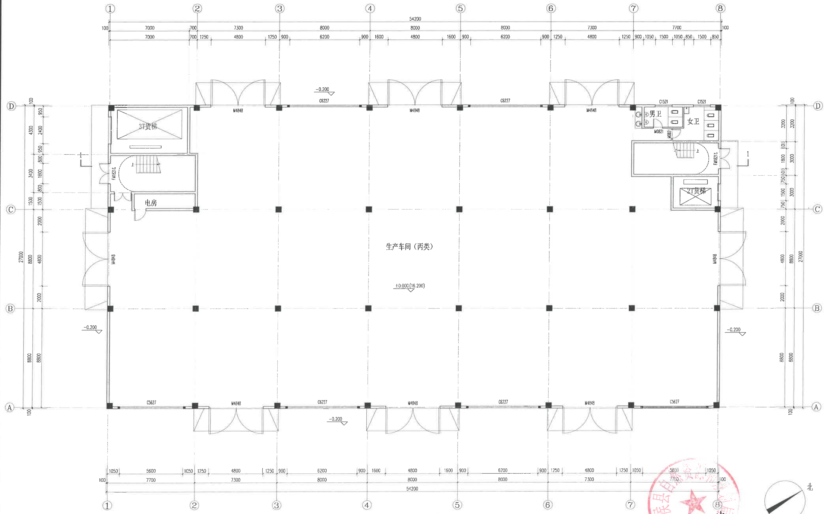
一层平面图 1:100
