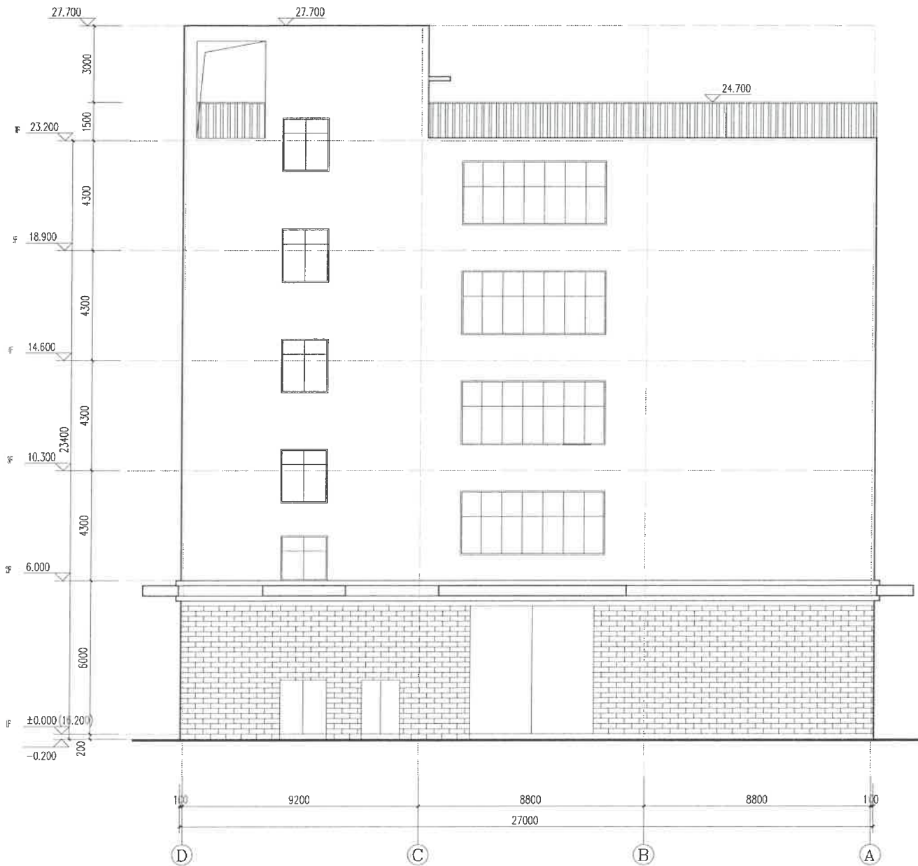
④-①轴立面图 1:100
