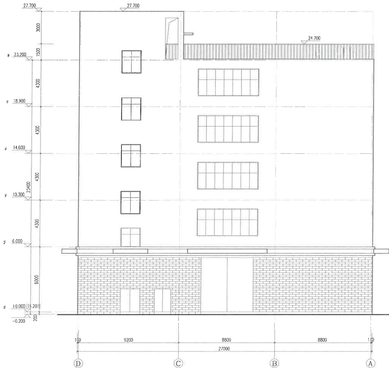
D-A轴立面图 1:100
