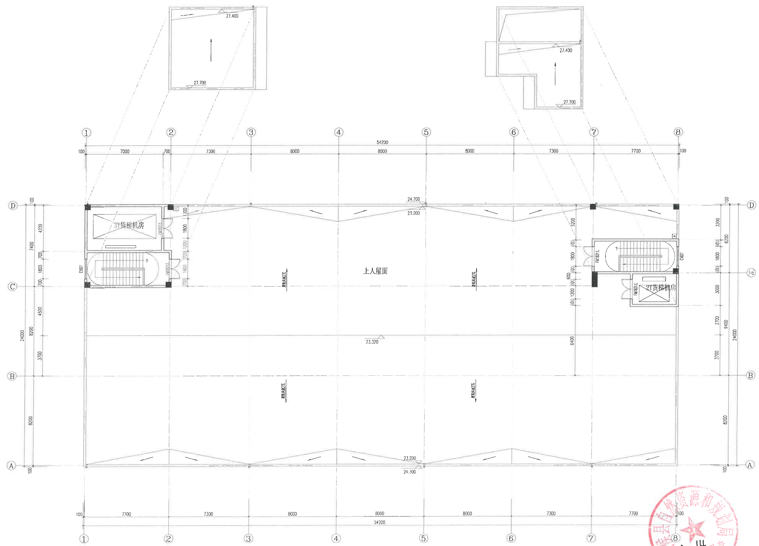
屋顶层平面图 1:100
