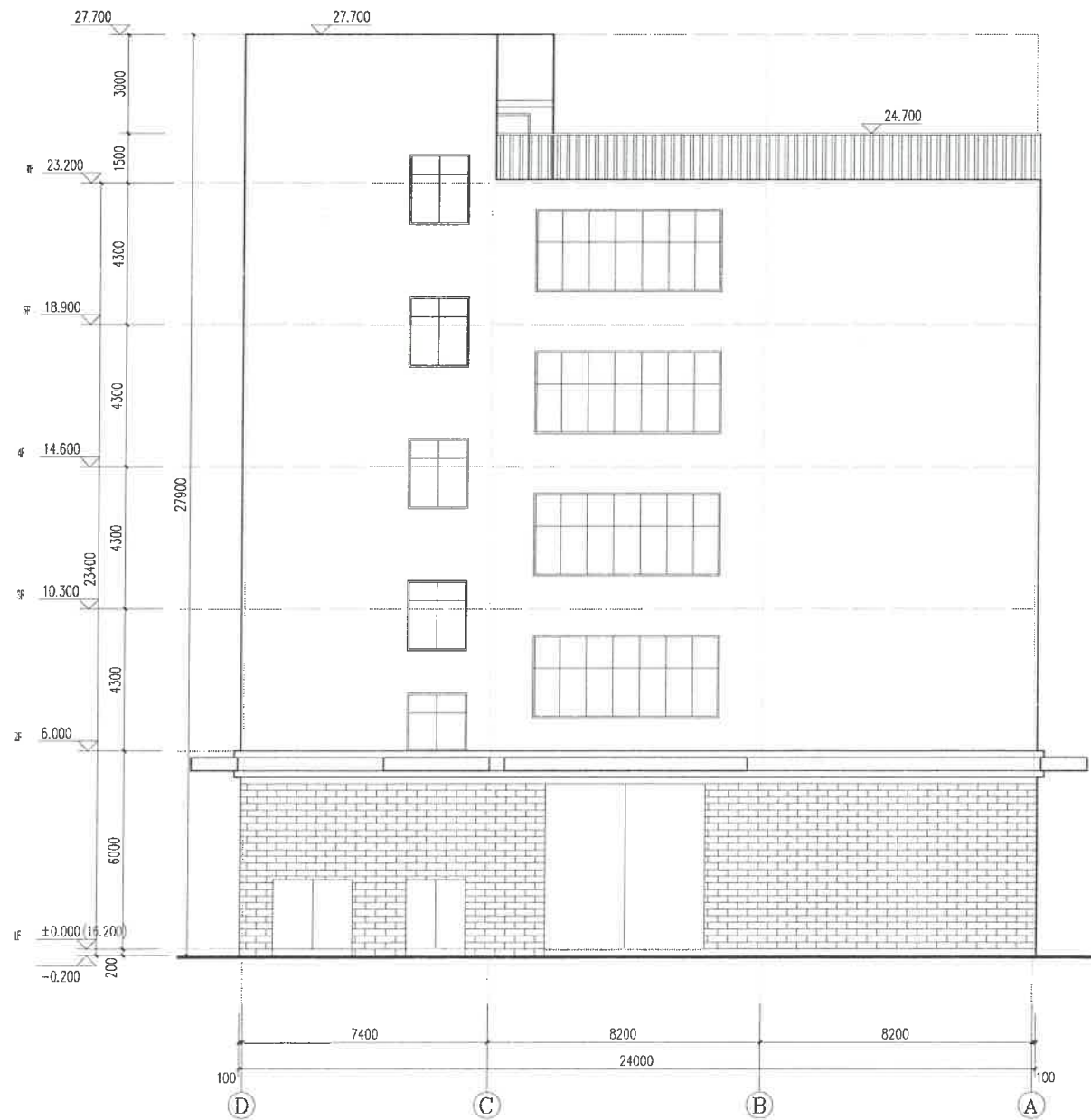
④-①轴立面图 1:100
