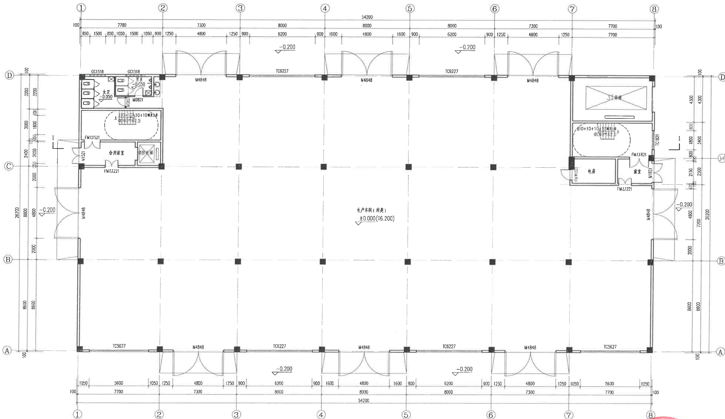
一层平面图 1:100
