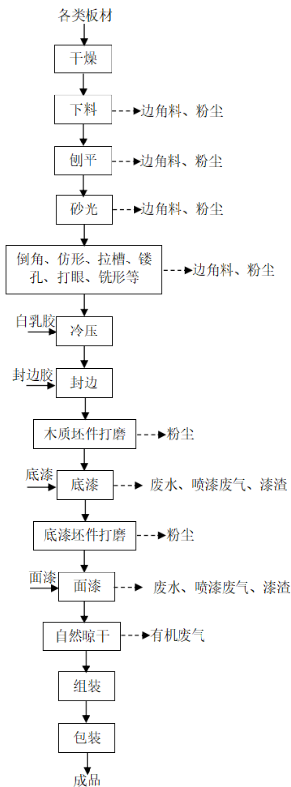
图 2-2 生产工艺流程图
