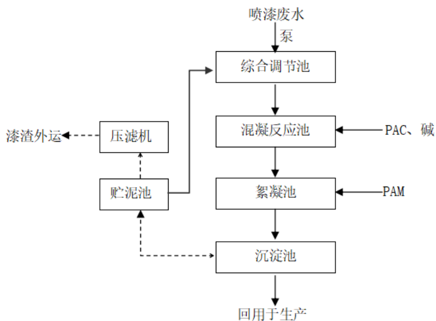
图 4.2-1 喷漆废水处理工艺流程图
