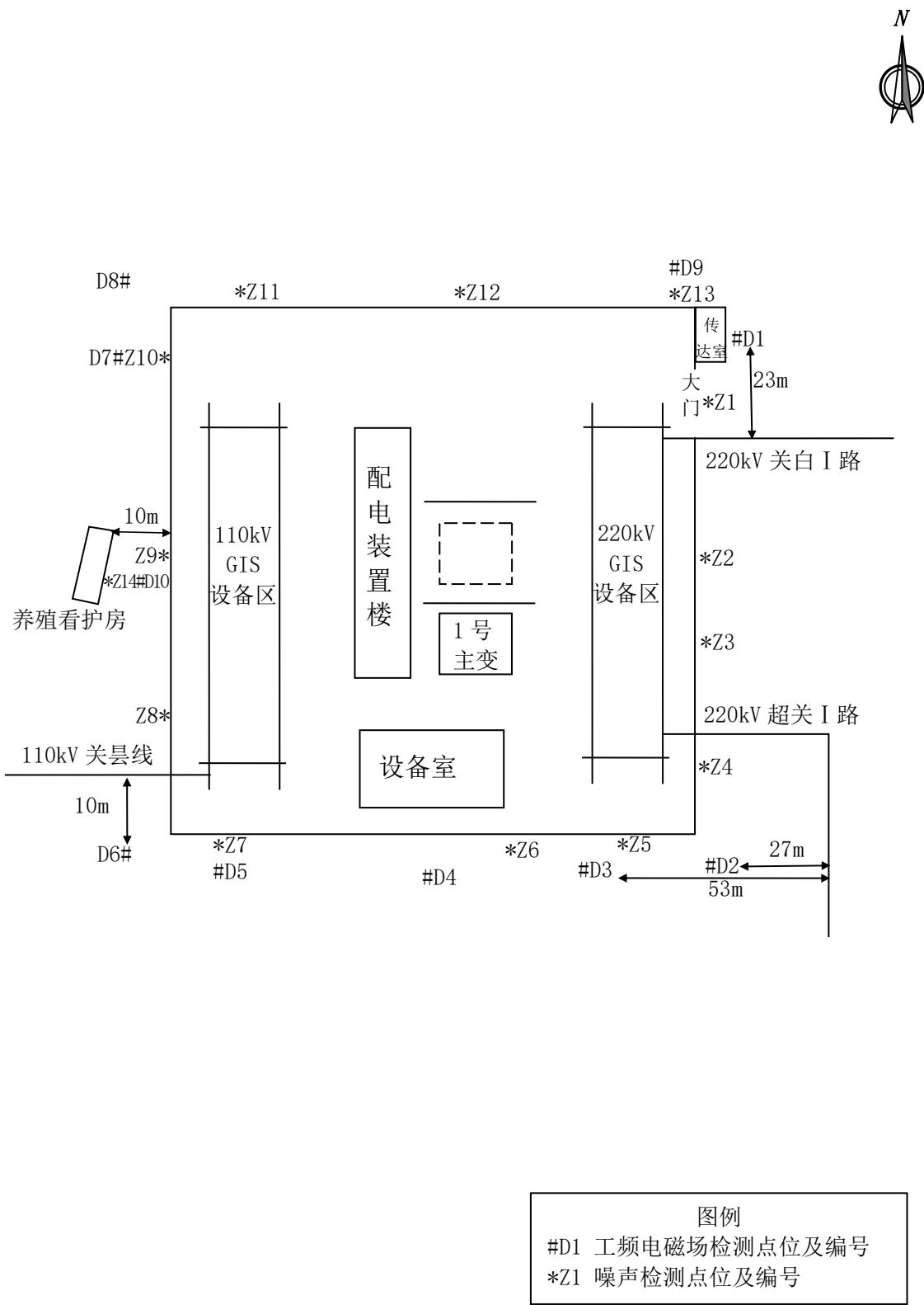
图 A-1 拟建福建福州关西 220kV 变电站主变扩建工程周围工频电场、磁感应强度、噪声测点布置示意图
