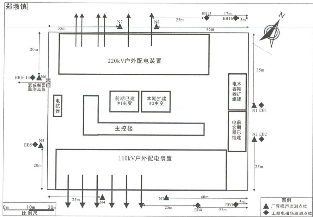
图 A-2 南平九龙 220kV 变电站平面布置及工频电场、工频磁场监测点位示意图
