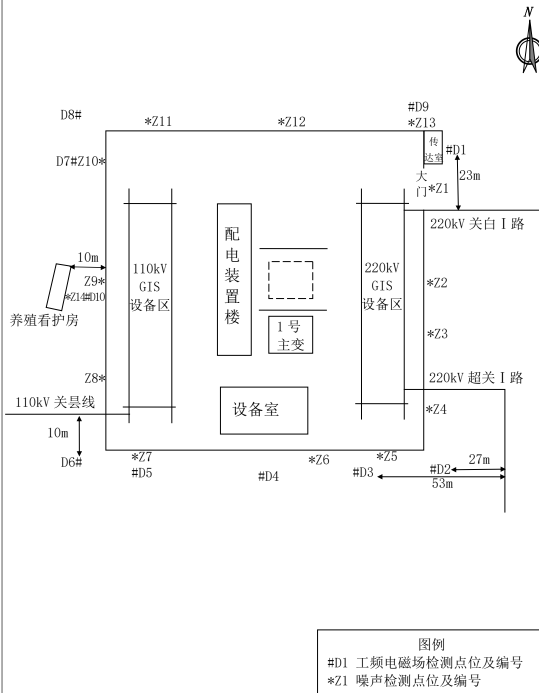
图 拟建福建福州关西 220kV 变电站主变扩建工程 (2 号主变) 周围工频电场、磁感应强度、噪声测点布置示意图
