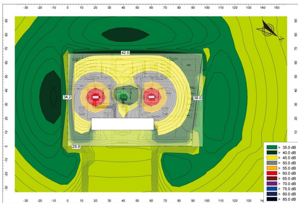
图 4-4 青洲 110kV 变电站等声值线图（终期）
