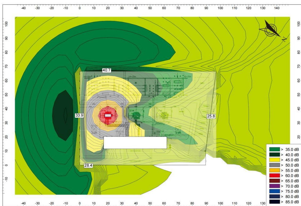
图 4-3 青洲 110kV 变电站等声值线图（本期）
