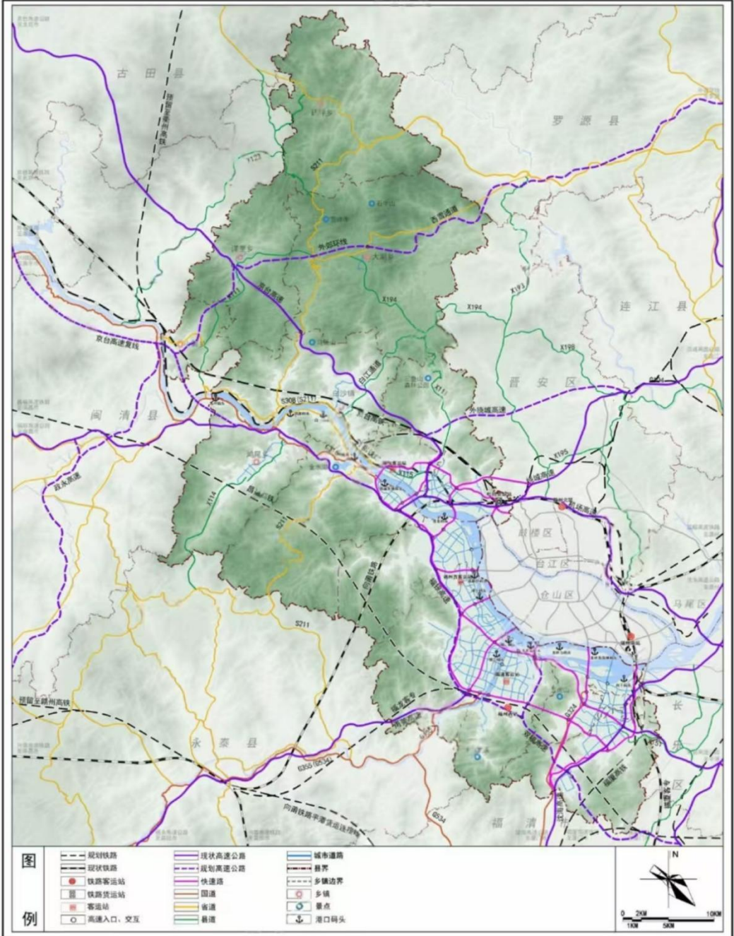
县域综合交通体系规划图
