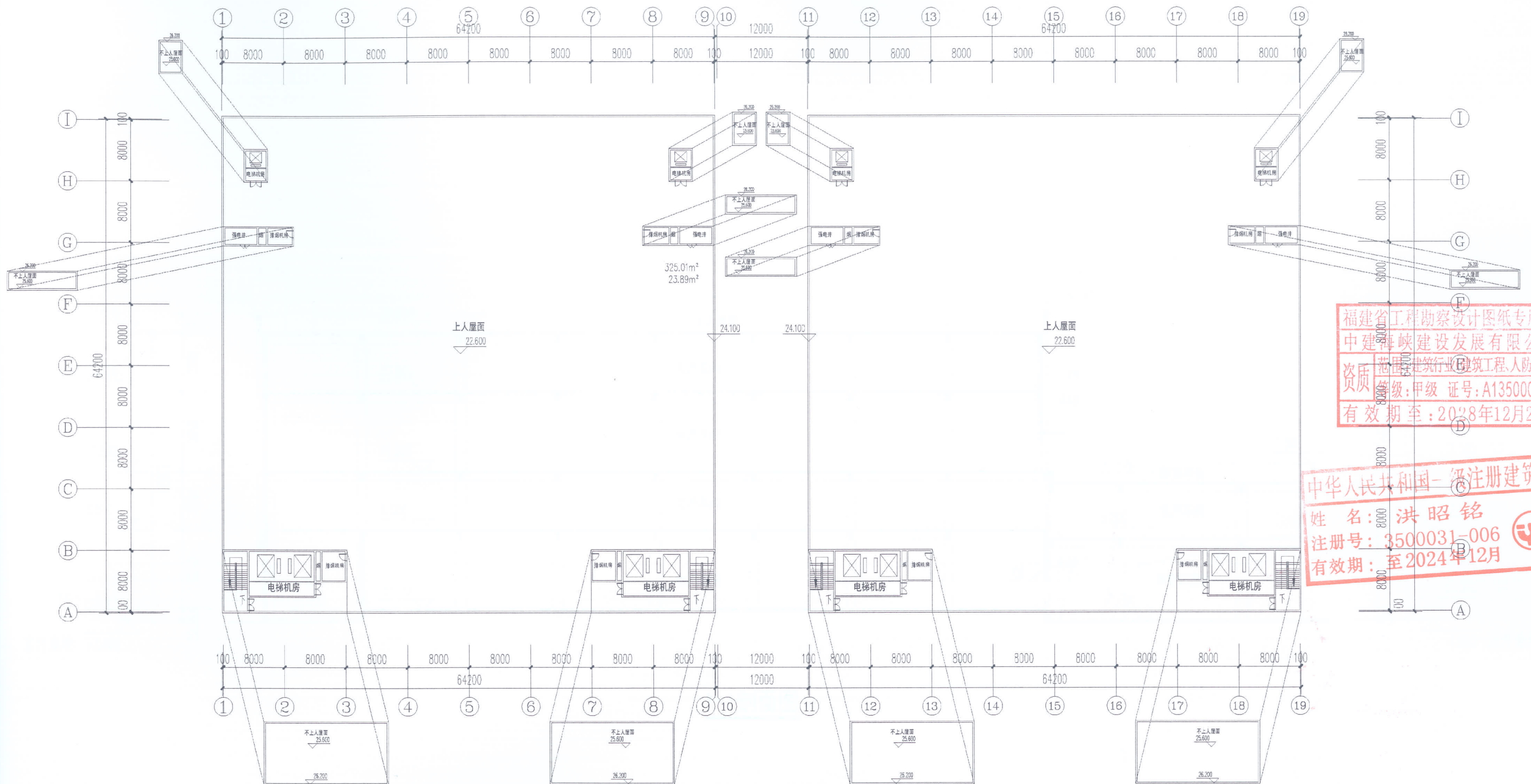
1#厂房屋面平面图
