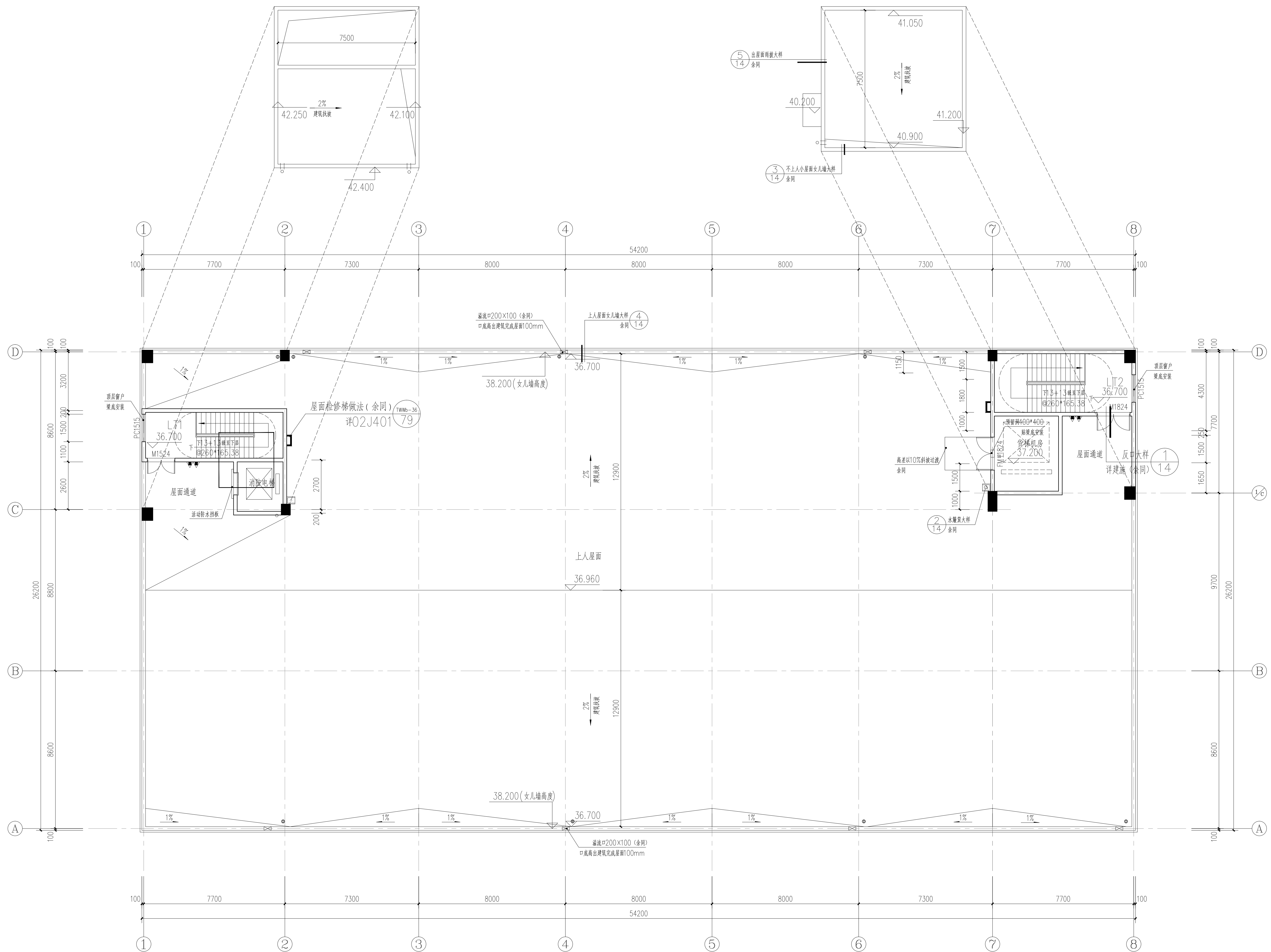
屋面层平面图 1:100
