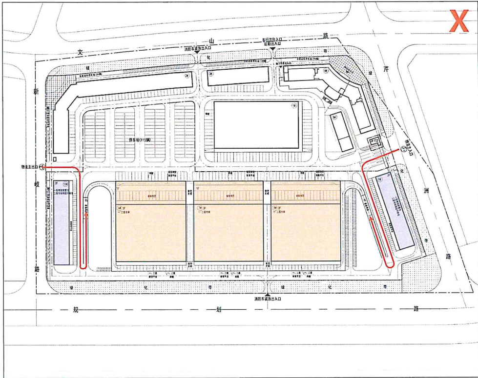
强排方案1
