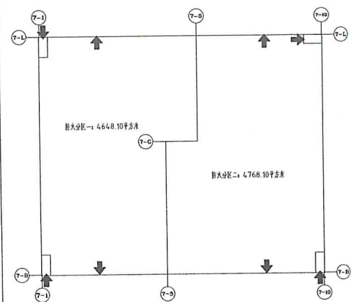
二层防火分区示意图
