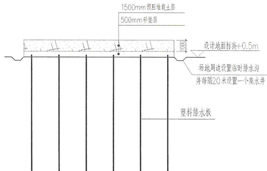
堆载预压做法示意图
