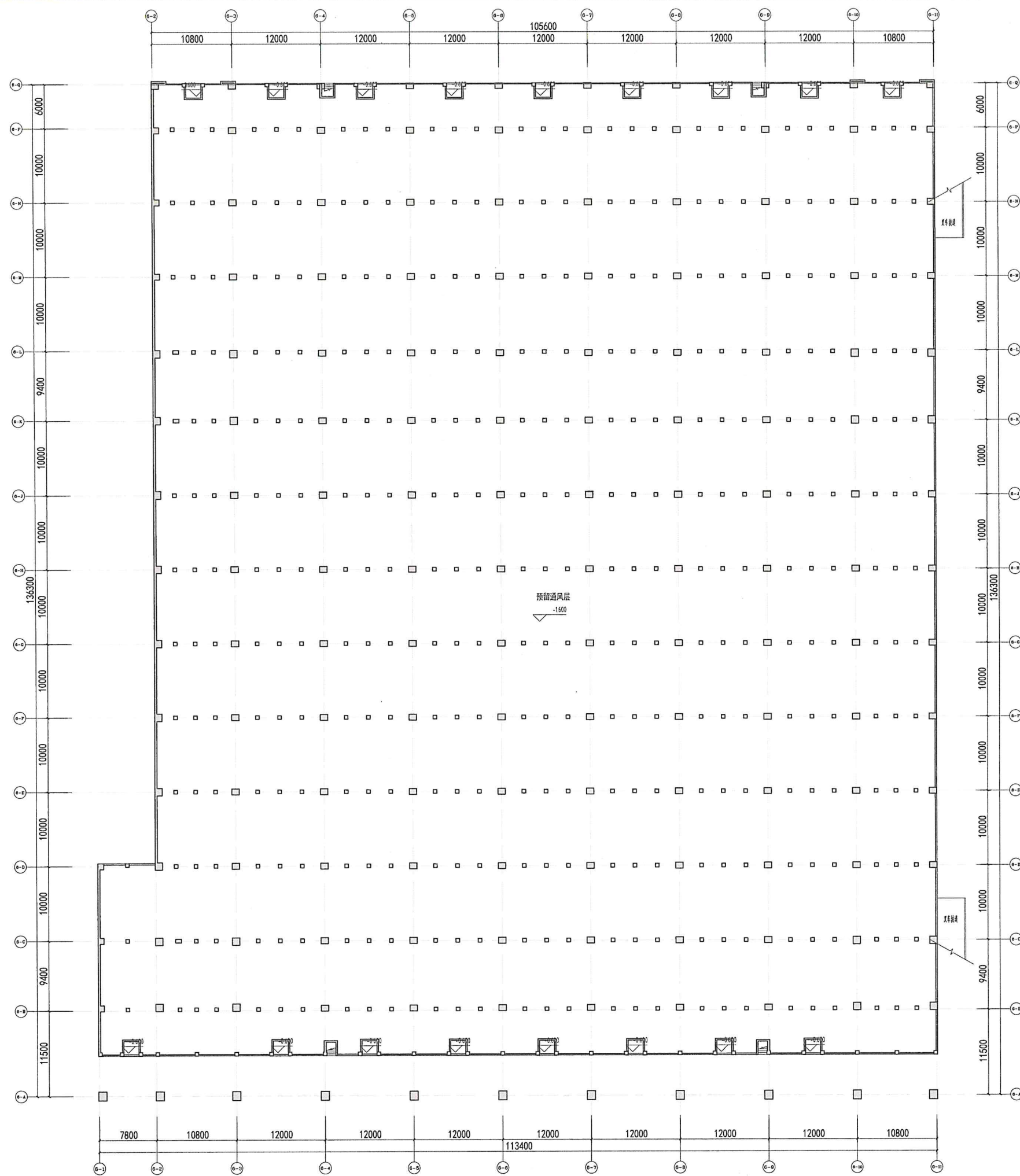
预留通风层平面图
