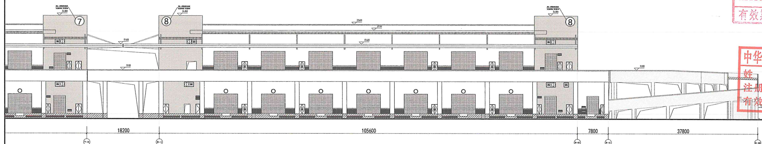
8-1轴~8-16轴立面图
