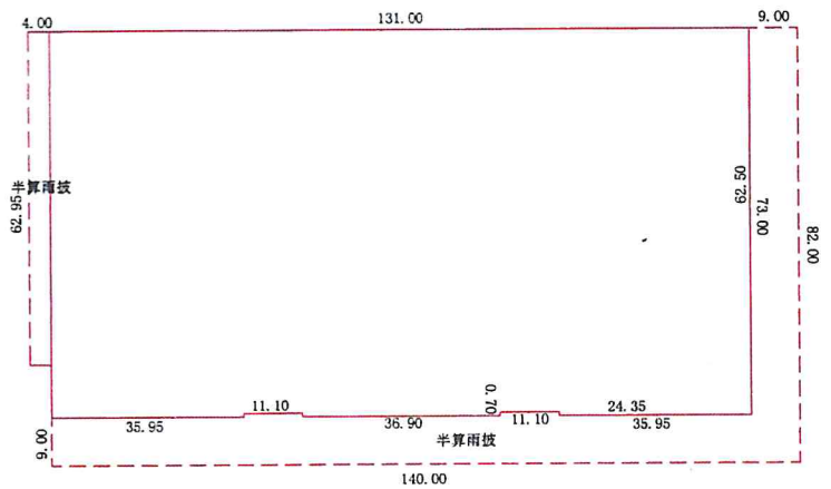
一层平面图
