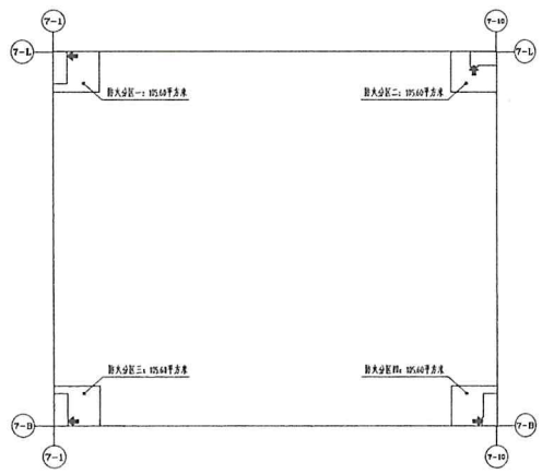
二层夹层防火分区示意图
