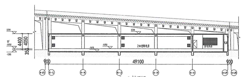
2-2剖面图 1:200
