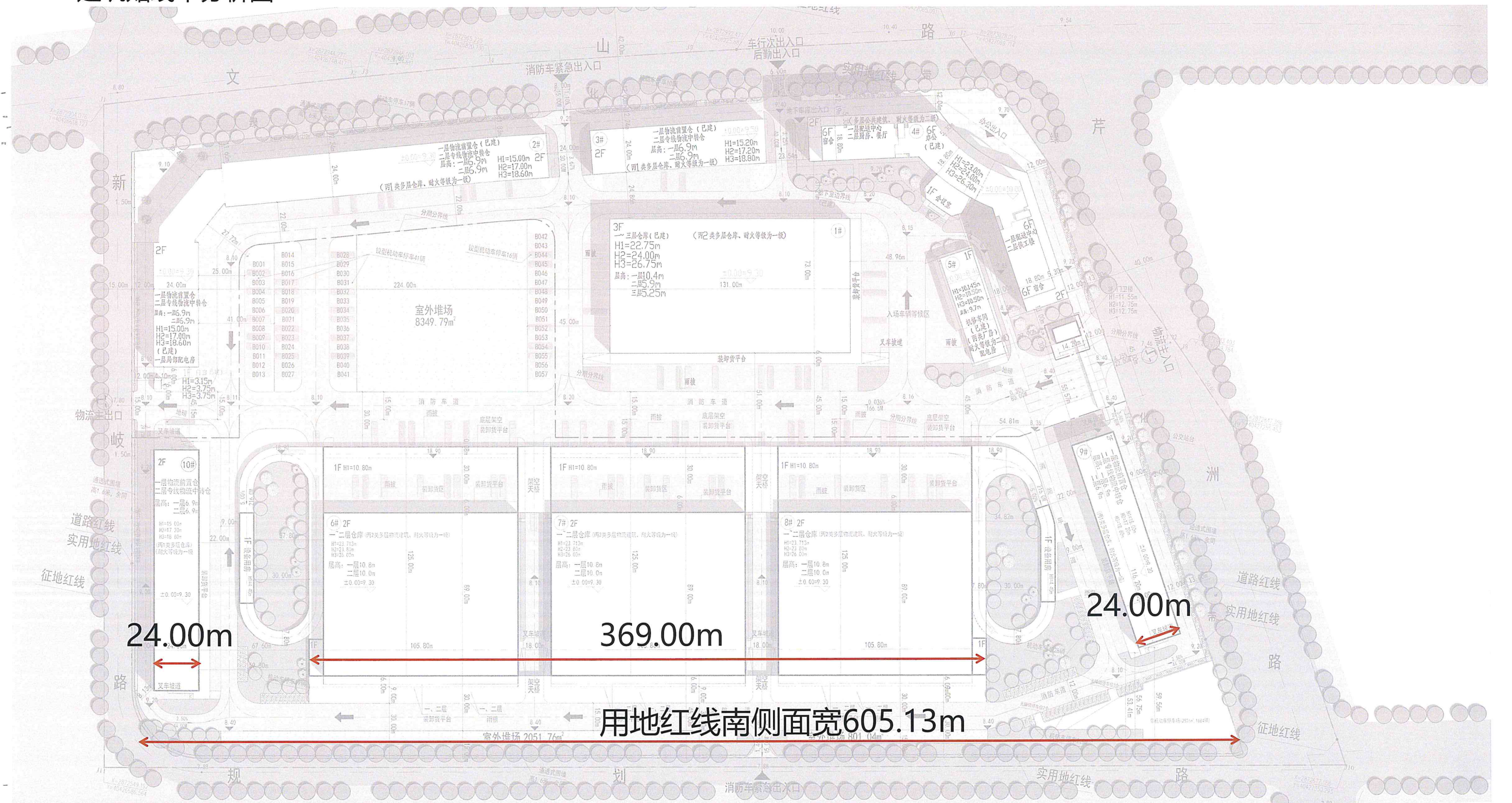
建筑贴线率分析图
