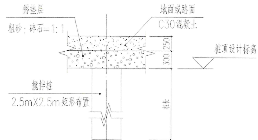
地面、路面搅拌桩剖面
