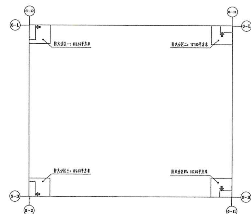
二层夹层防火分区示意图
