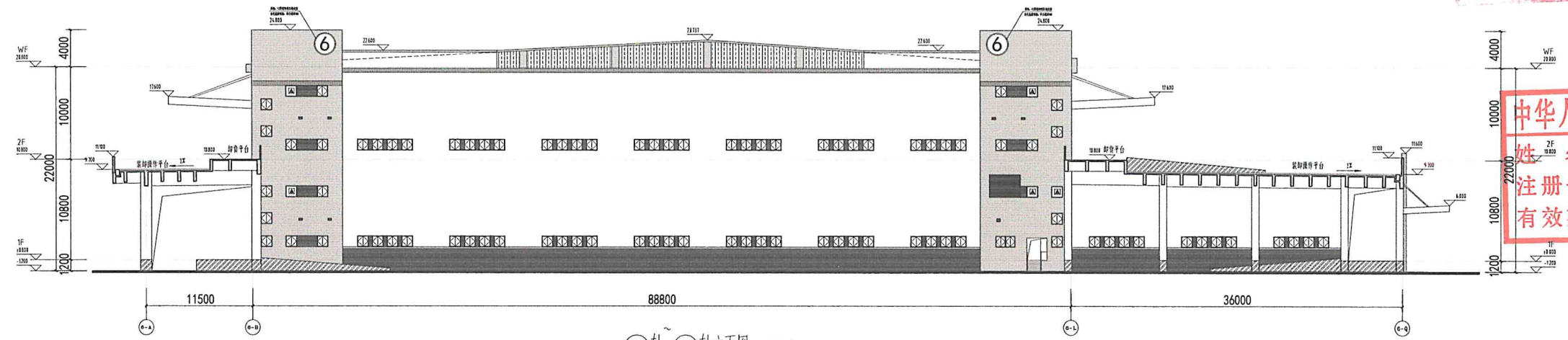
6-A~6-D轴立面图 1:200
