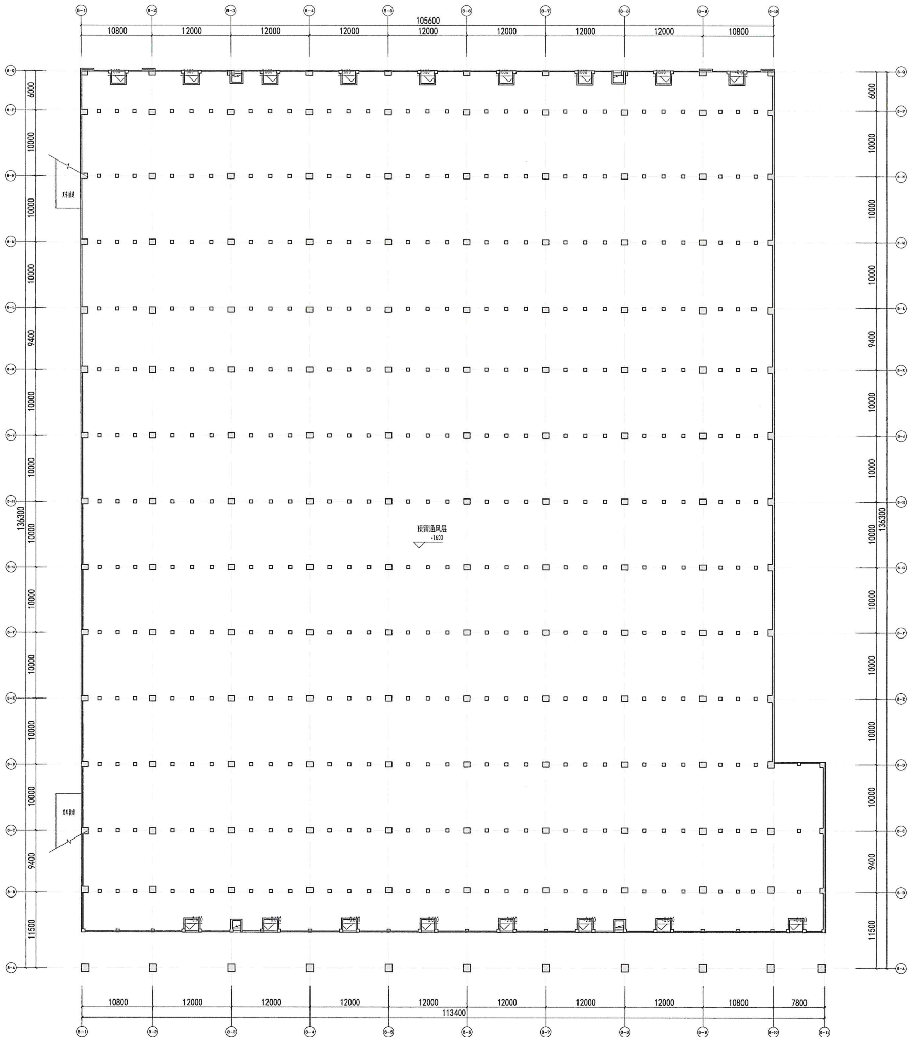
预留通风层平面图
