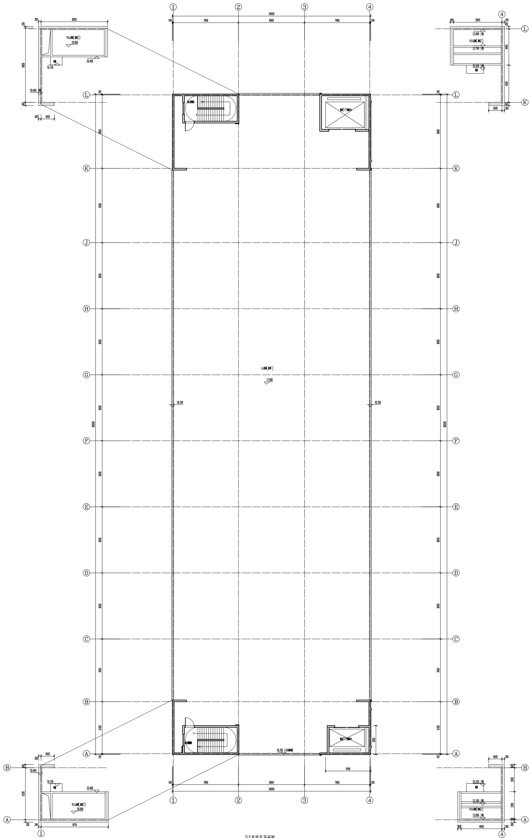
9#屋顶层平面图 1:100
