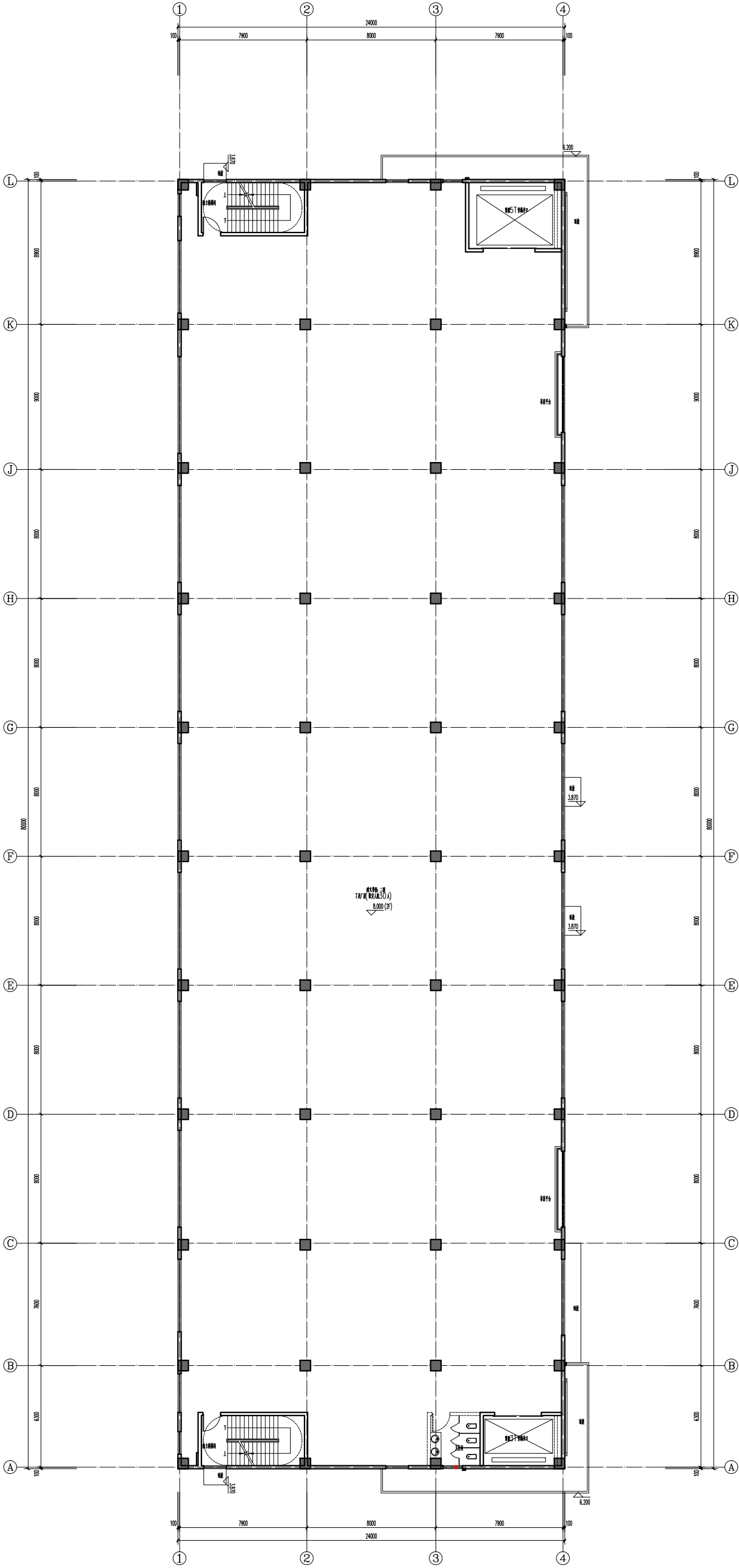
9#二层平面图 1:100
