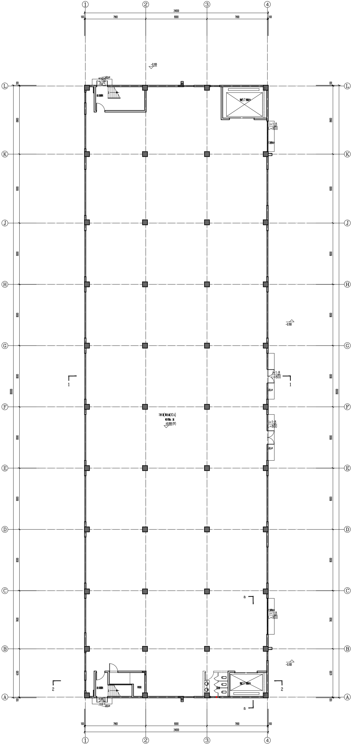
9#一层平面图 1:100
