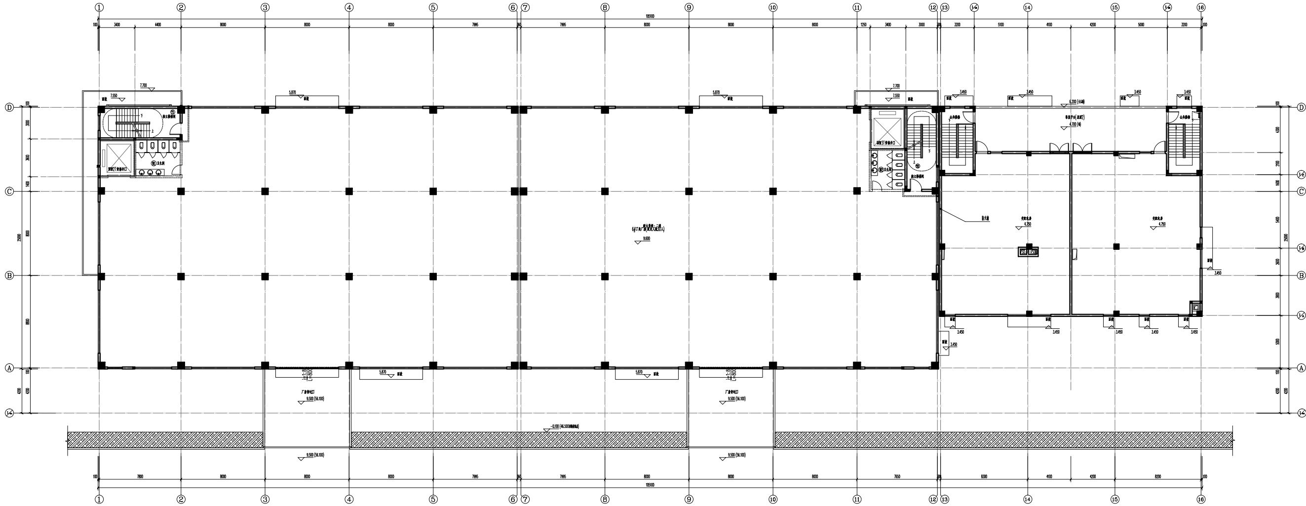
6#二层平面图 1:100 6#楼层建筑面积: 2004.20m 2 6#楼层计容面积: 2004.20m 2
