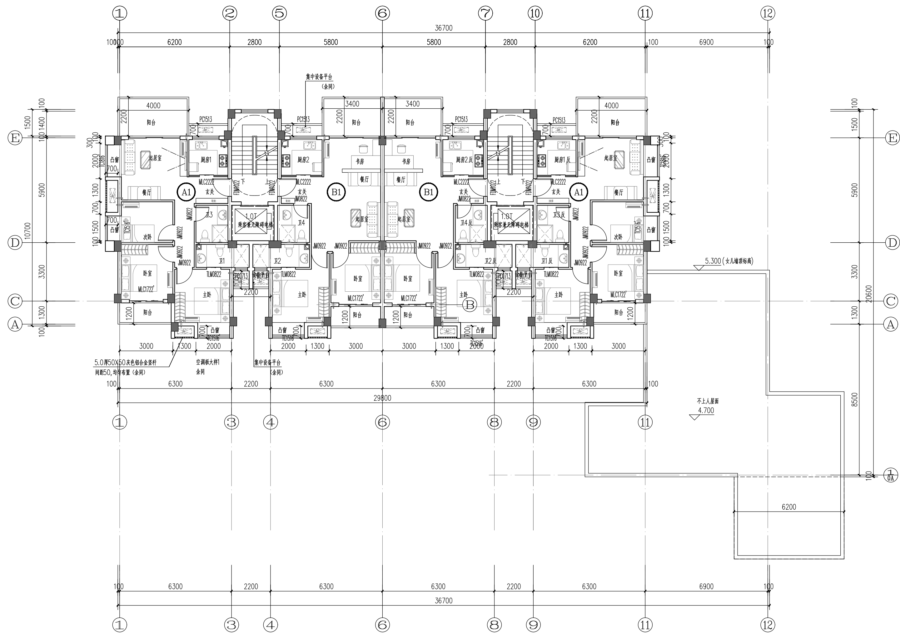
2#楼二层平面
