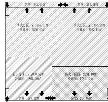
二层防火分区示意图
