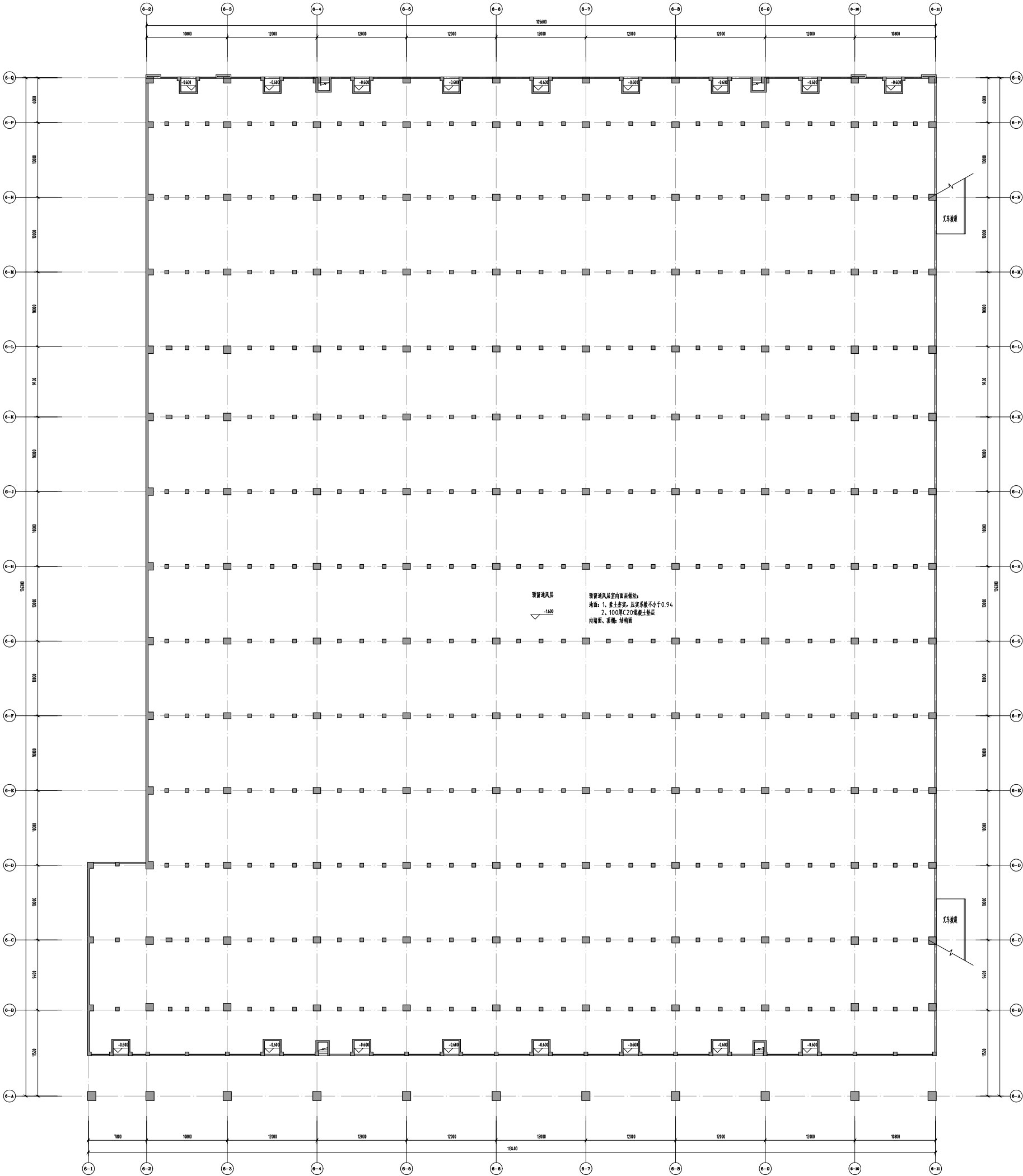
预置通风层平面图 1:200
