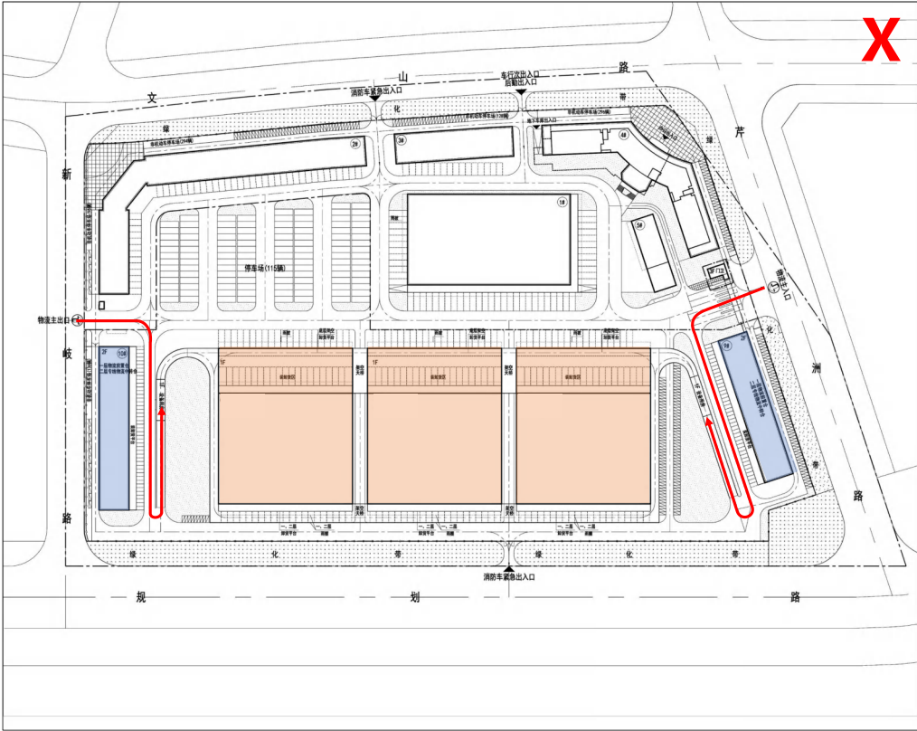
强排方案1
