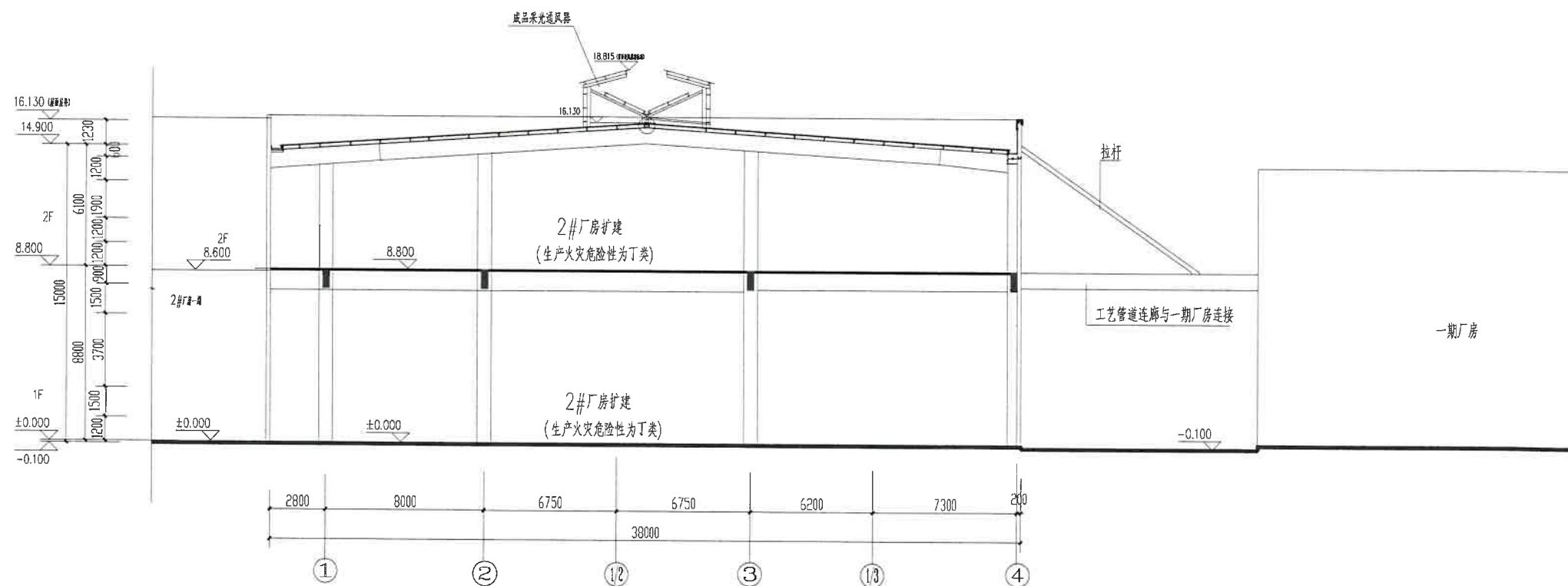
I-I剖面图 1:150
