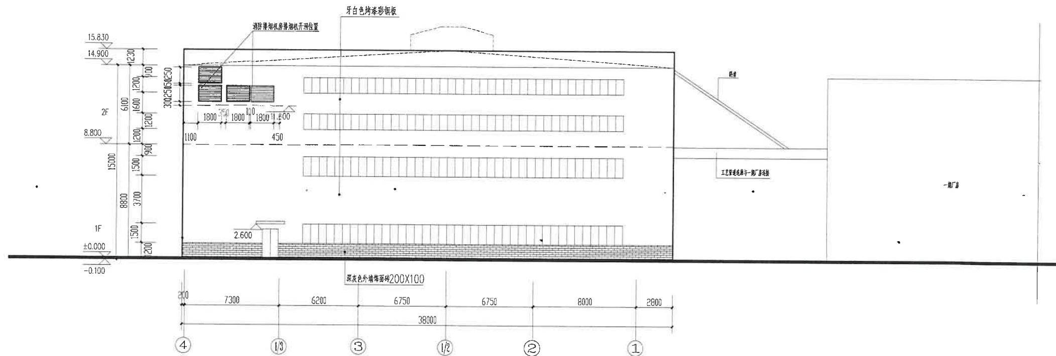
④-①立面图 1:150
