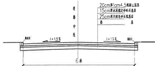
厂区道路横断面图
