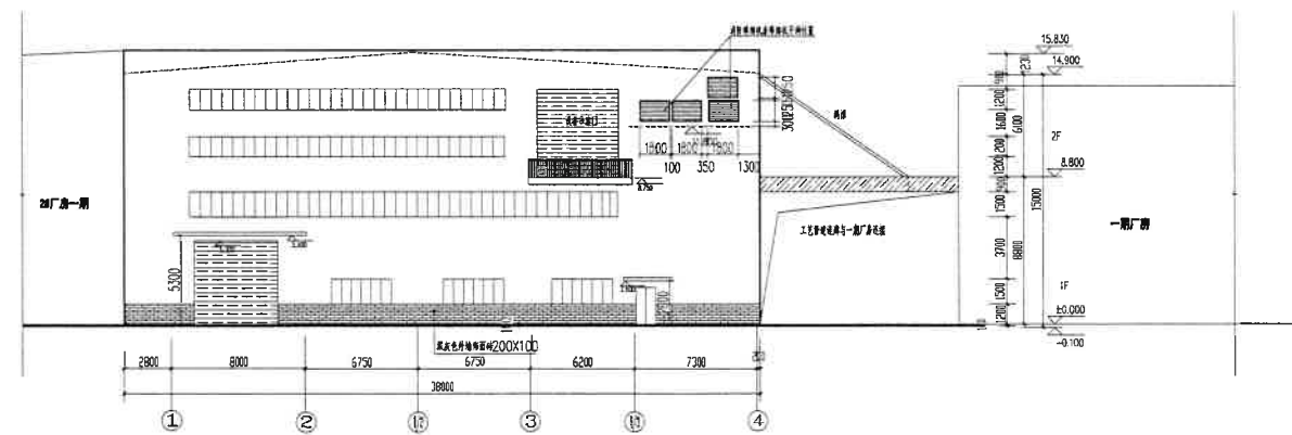
①-④立面图 1:150
