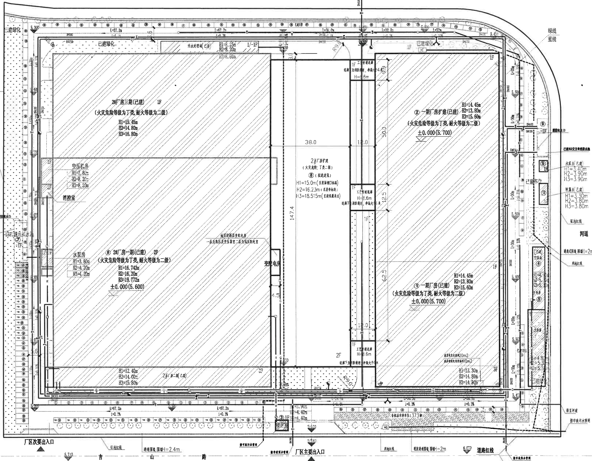
室外管线综合总平面图 1:500
