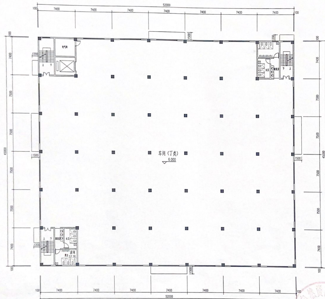
二层平面图
