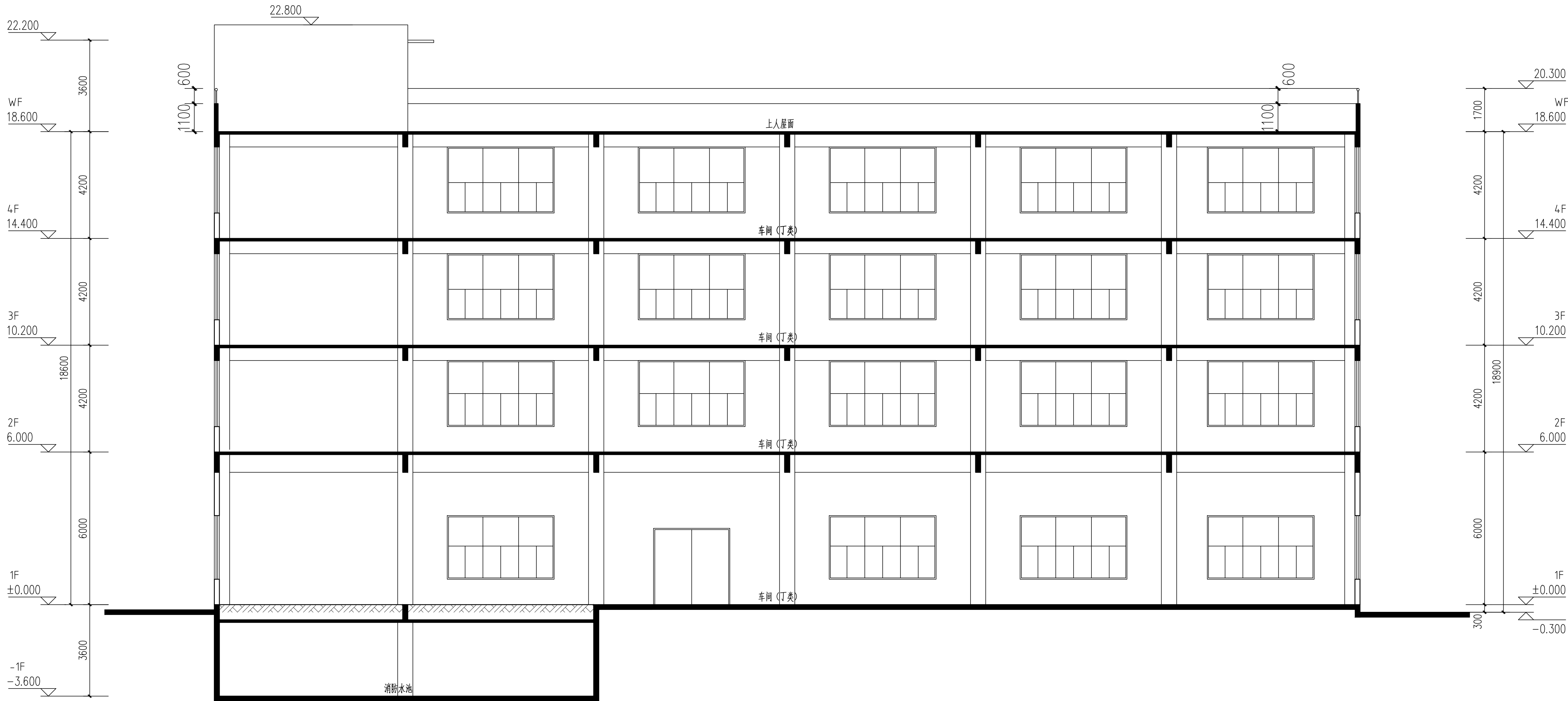
1-1剖面图
