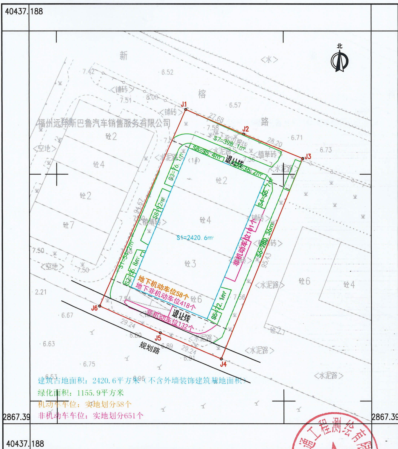
建筑占地、绿化面积略图
